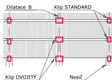
Obr. 6 Napojování terasových prken pomocí DVOJITÉHO KLIPU
